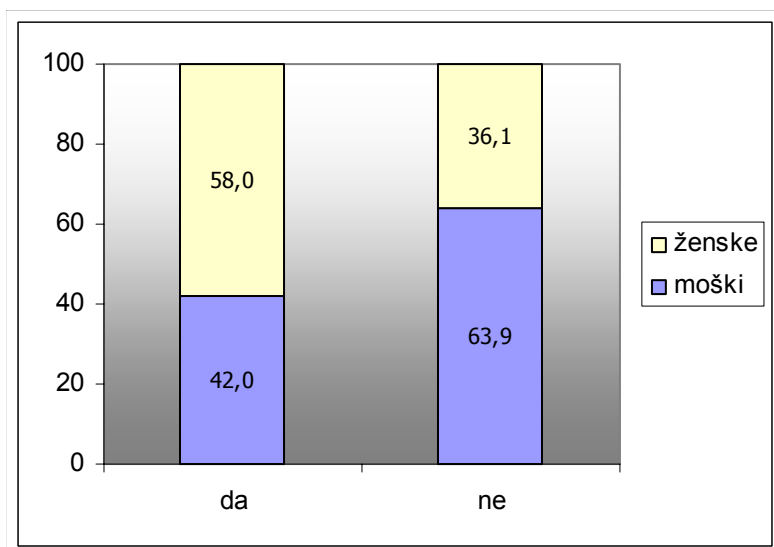
Graf 10: Ali menite, da je ena klobuta nasilno ravnanje glede na spol respondentov (v %):
