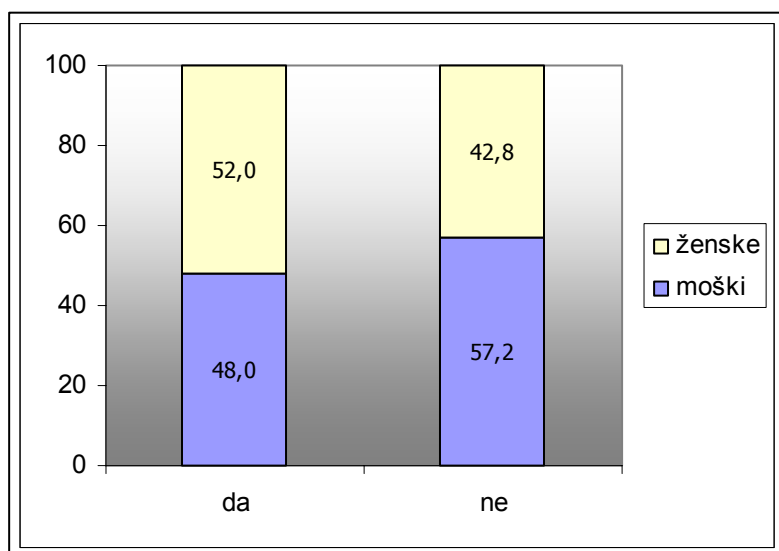
Graf 12: Ali menite, da je grožnja nasilno ravnanje glede na spol respondentov (v %):
