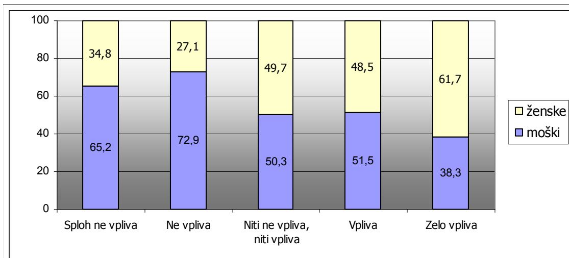
Graf 17: Ali menite, da nezadovoljstvo s partnerskim življenjem vpliva na nasilje v družini glede na spol respondentov (v %):
