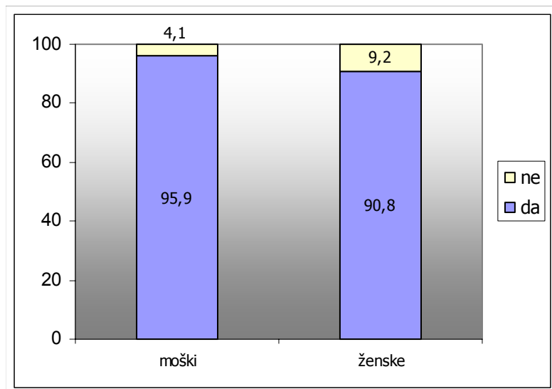
Graf 18: Ali veste, da je prisila partnerke v spolni odnos kaznivo dejanje glede na spol respondentov (v %):
