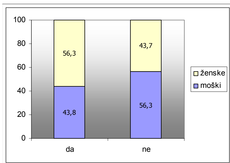
Graf 11: Ali menite, da je pregledovanje žepov nasilno ravnanje glede na spol respondentov (v %):
