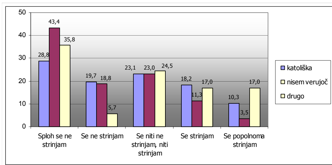
Graf 22: Intelektualno delo je bolj primerno za moške glede na veroizpoved respondentov (v %):
