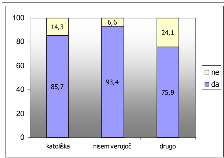
Graf 14: Ali menite, da je verbalno poniževanje nasilno ravnanje glede na veroizpoved respondentov (v %):
